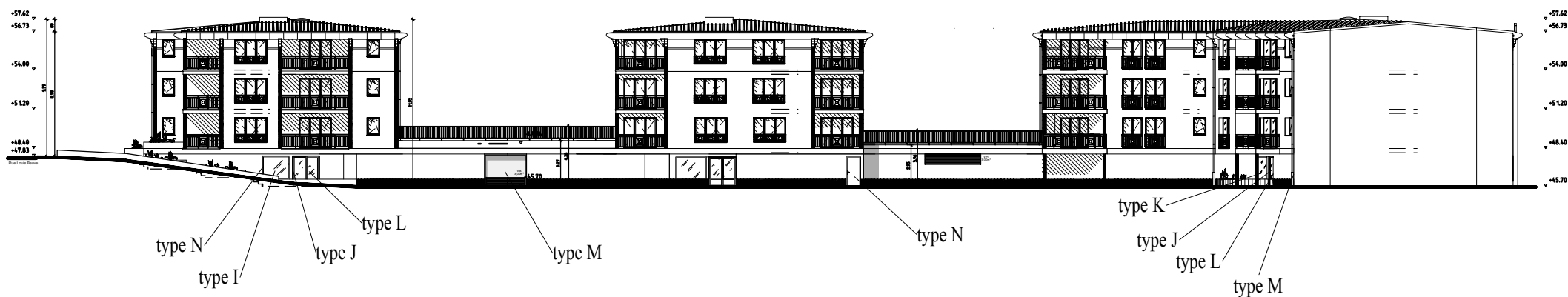
Façade Ouest
